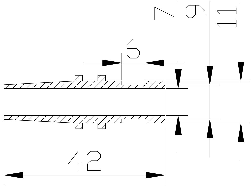
Sezione A-A
